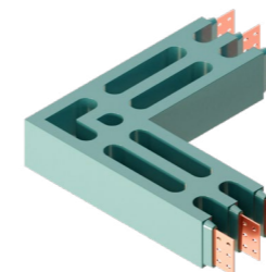
Угол горизонтальный
